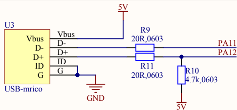
USB电路
