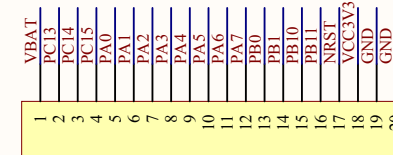
P3 Header 20
